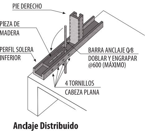
Barra de Anclaje o Espárrago AN2
