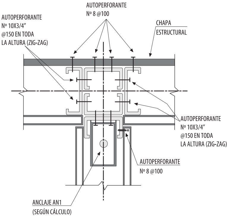
Encuentro centro (T)
